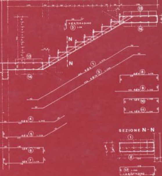
SEZIONE SCHEMATICA DI RIFERIMENTO
