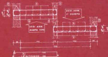
SEZIONE TRASVERSALE S · S
